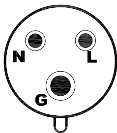
IEC60309 32A
